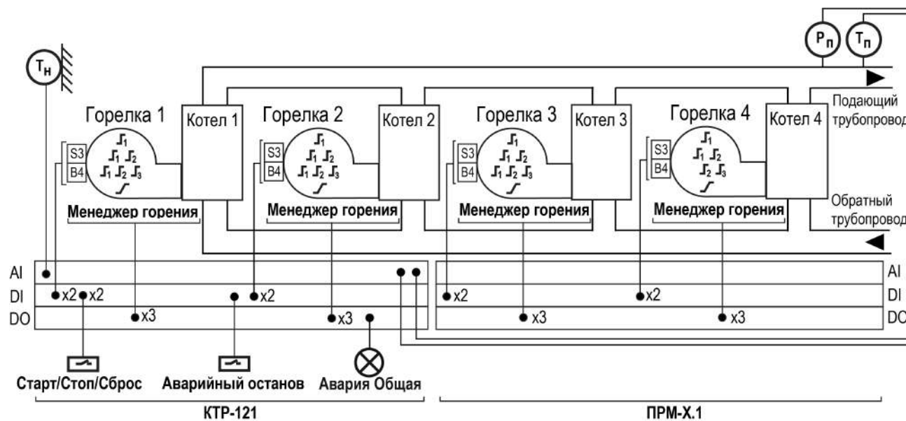
Рисунок 1.1 – Объект управления
