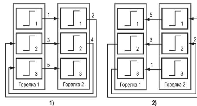
Рисунок 10.4 – Регулирование температуры по «1122»: 1) включение, 2) выключение
