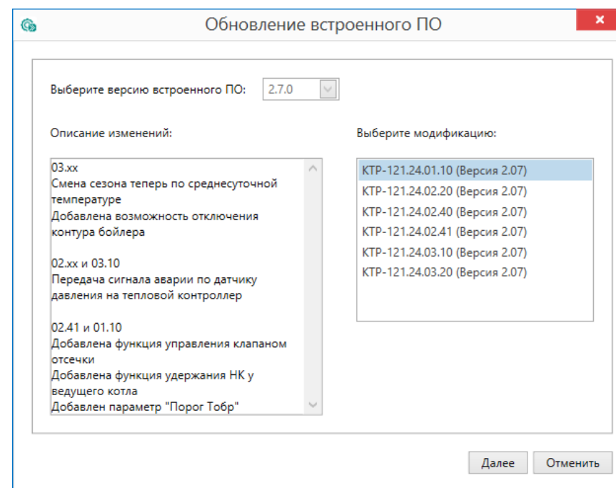
Рисунок 6.7 – Выбор алгоритма
